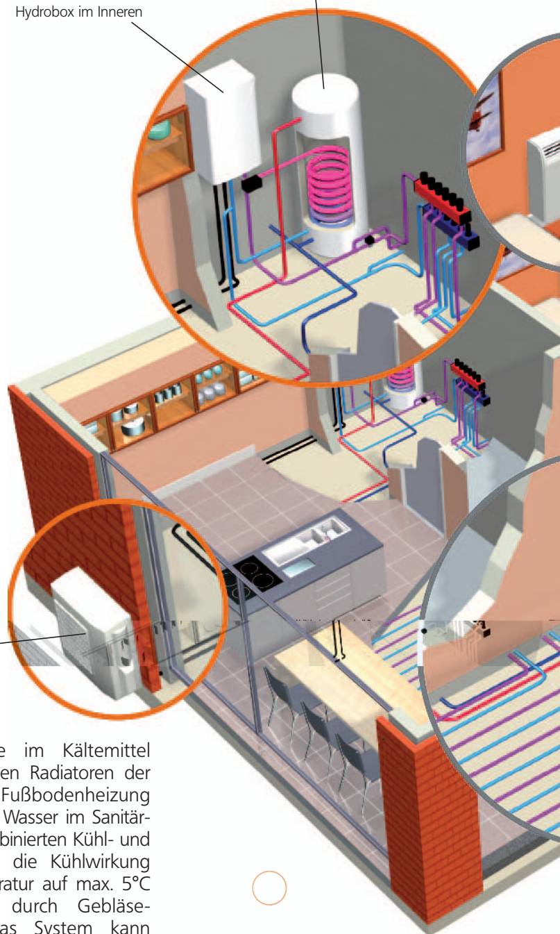
Hydrobox im Inneren
